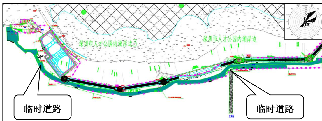
图 2.4-3 临时道路布置图
