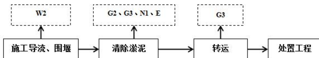
图 3.1-3 清淤工程施工工艺及产污环节
