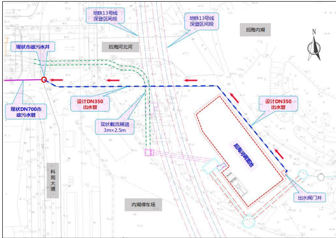
图 2.5-7 调蓄池出水方案平面图
